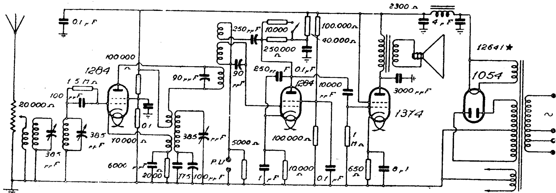
WATT RADIO - MOD. « TELEDINA »
